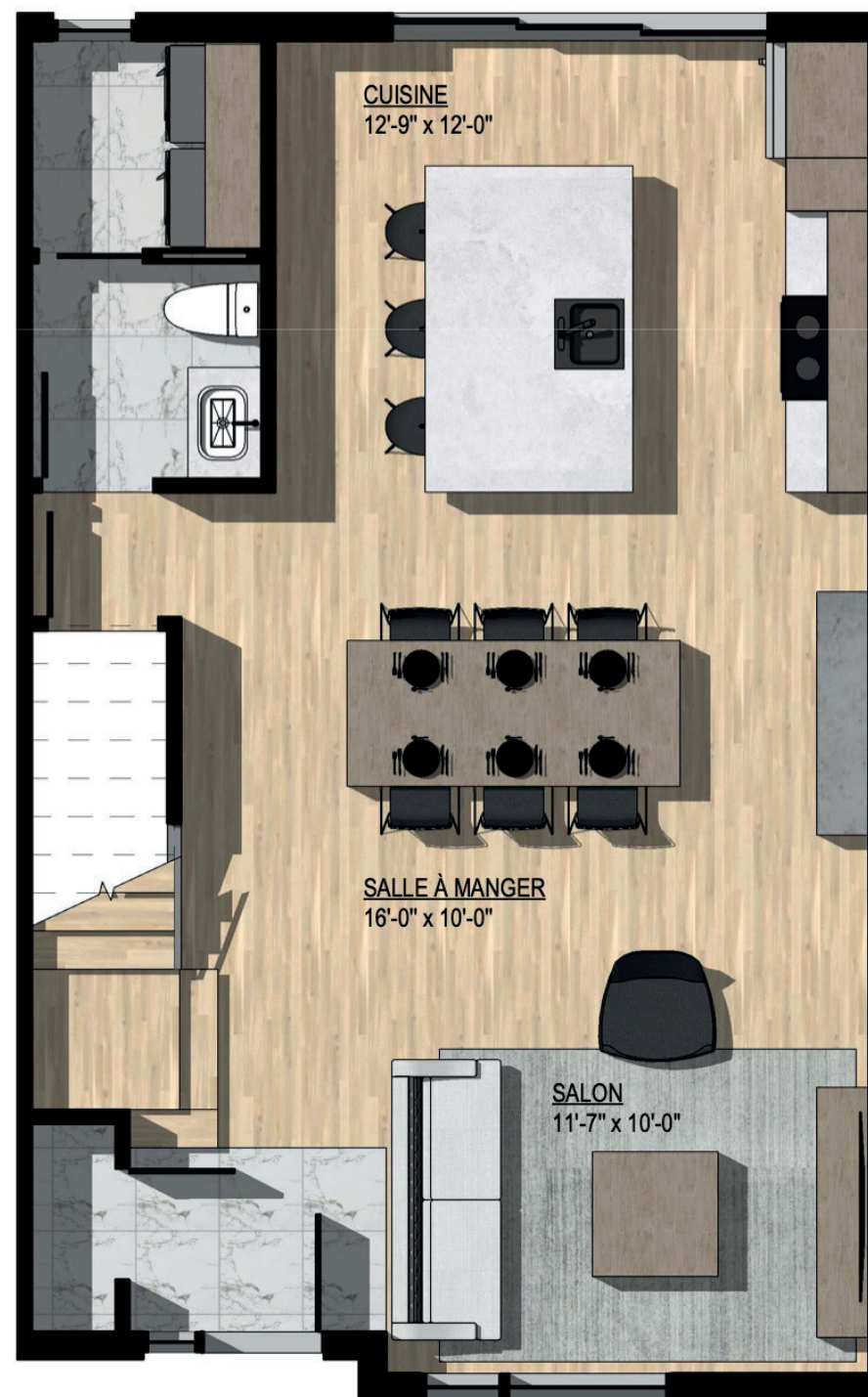
REZ-DE-CHAUSSÉE – 700 PI²
